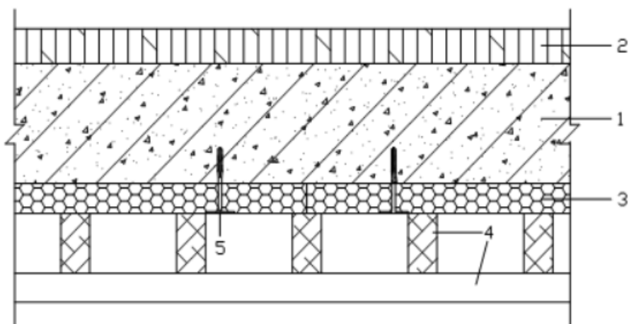
1-混凝土墙体；2-无需保温一侧普通模板及支撑；3-保温板；4-TCC 保温模板支架；5-锚栓
